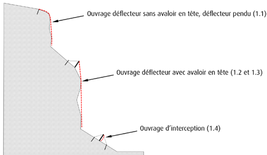
Figure 1 : Principe général des ouvrages déflecteurs (Source : C2ROP)
